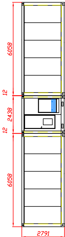
POGLEĐ "B"
