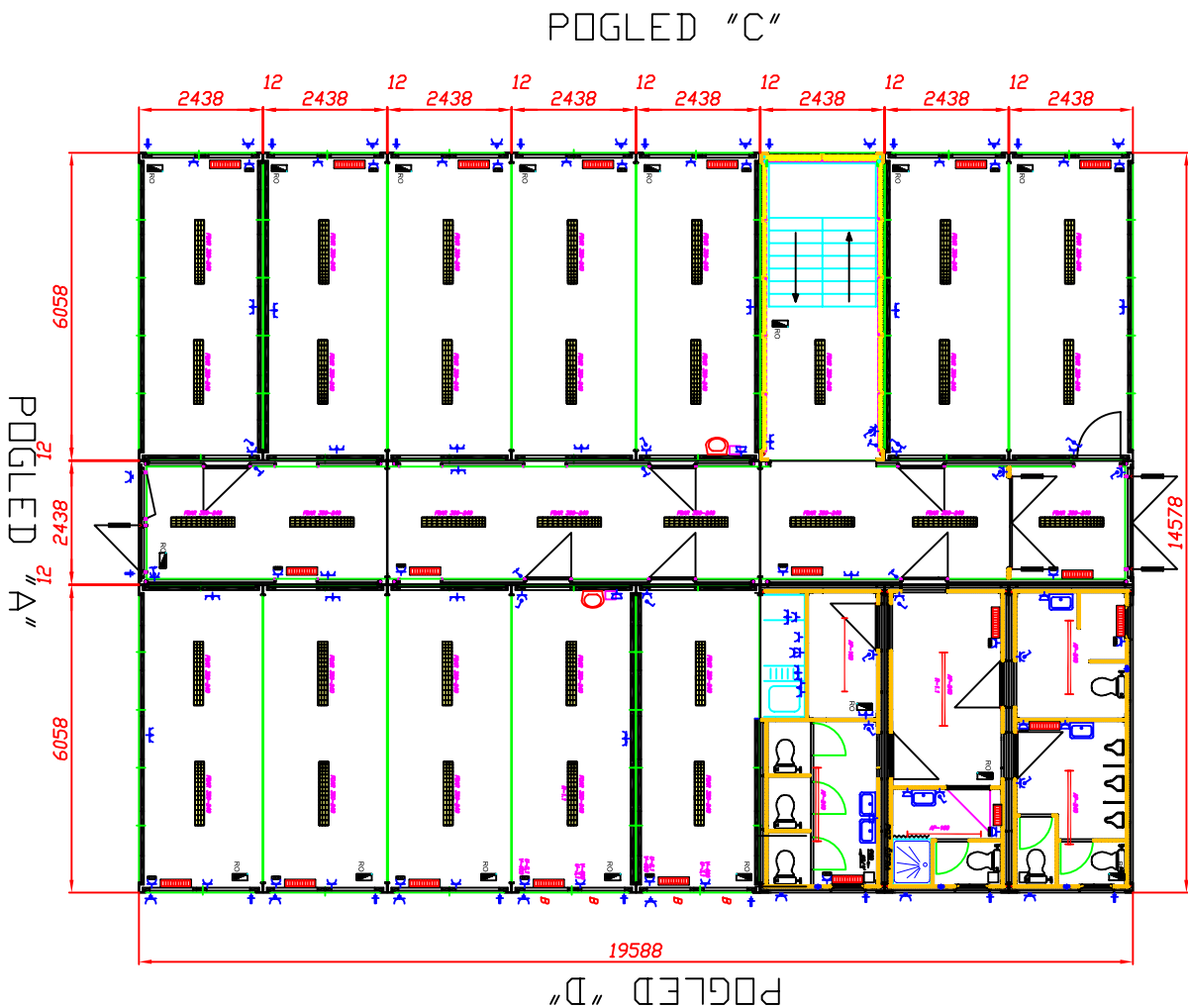
POGLEĐ "A"
