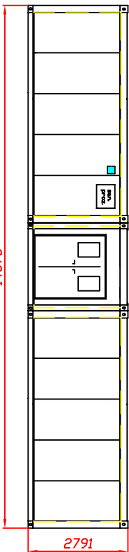
POGLEĐ "B"
